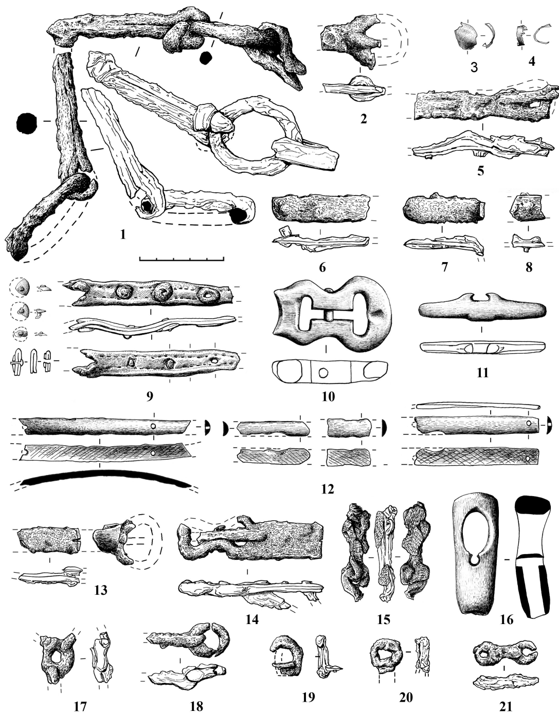
Рис. 4. Снаряжение верхового коня и человека из погребения кургана № 30а некрополя Чобурак-I (рисунки выполнены И.А. Чудилиным):
